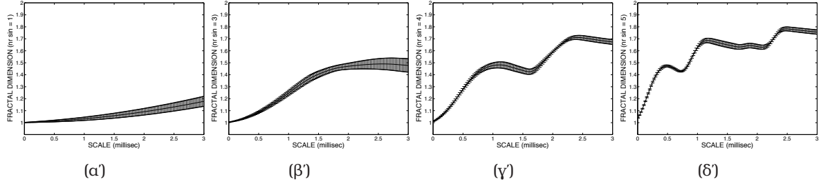
Σχήμα 3.8: Μέση τιμή του MFD και τυπική απόκλιση συνθετικών ημιτονοειδών σημάτων. (α') Αρχικό ημίτονο x_0 = x_{50} (50 Hz), (β') x = x_{50} + x_{100} + x_{200} , (γ') x = x_{50} + x_{100} + x_{200} + x_{400} και (δ') x = x_{50} + x_{100} + x_{200} + x_{400} + x_{800} .
