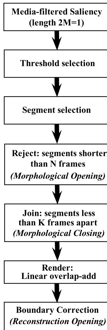
Σχήμα 5.5: Αλγόριθμος δημιουργίας ηχητικών περιλήψεων μετά τη σύμμιξη.
