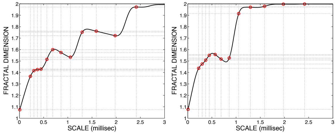
Σχήμα 3.12: Παράδειγμα των δεκατριών λογαριθμικά επιλεγμένων σημείων του MFD για τη νότα A3 του B \flat κλαρινέτου και τη νότα A4 για το φαγκότο, τα οποία δημιουργούν το σύνολο χαρακτηριστικών MFDLG.
