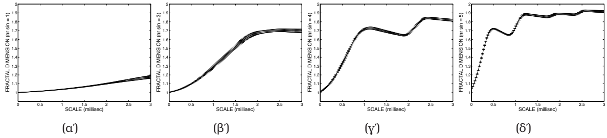
Σχήμα 3.9: Μέση τιμή του MFD και τυπική απόκλιση συνθετικών ημιτονοειδών σημάτων ενώ προστίθενται ημίτονα διπλάσιας συχνότητας με πλάτος το οποίο μειώνεται γεωμετρικά. (α') Αρχικό ημίτονο x_0 = x_{50,1} (όπου 50 σε Hz και 1 το πλάτος), (β') x = x_{50,1} + x_{100,1/2} + x_{200,1/4} , (γ') x = x_{50,1} + x_{100,1/2} + x_{200,1/4} + x_{400,1/8} , και (δ') x = x_{50,1} + x_{100,1/2} + x_{200,1/4} + x_{400,1/8} + x_{800,1/16} . Η φάση μεταβάλλεται με τυχαίο τρόπο.
