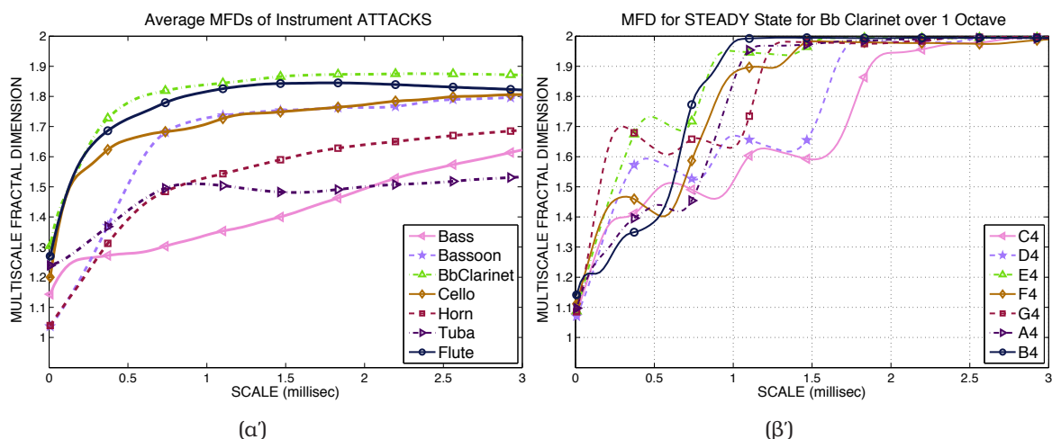
Σχήμα 3.5: (α') Μέση τιμή του MFD προφίλ υπολογισμένη για το attack των επτά μουσικών οργάνων, και για όλο το εύρος συχνοτήτων (με χρήση παραθύρων ανάλυσης 30 ms). (β') MFD προφίλ για τη σταθερή κατάσταση τόνων μιας οκτάβας του Β \flat κλαρινέτου, για ένα παράθυρο των 30 ms.
