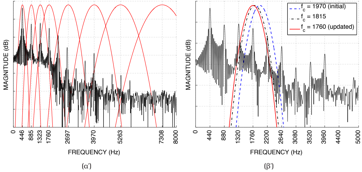
Σχήμα 4.1: (α') Συστοιχία φίλτρων Gabor (φίλτρα 2–9) με τις εκτιμώμενες κεντρικές συχνότητες f_c μετά την εφαρμογή του επαναληπτικού-ESA μαζί με το φάσμα της νότας A4 του Bb κλαρινέτου για ένα πλαίσιο ανάλυσης 30 ms ( F_s = 44.1 Hz). (β') Φάσμα της νότας A4 του Bb κλαρινέτου για ένα πλαίσιο ανάλυσης των 30 ms μαζί με το πέμπτο φίλτρο Gabor. Ο αλγόριθμος Iterative-ESA εφαρμόστηκε για το πέμπτο φίλτρο με αρχική κεντρική συχνότητα f_c = 1970 Hz και ύστερα από δύο επαναλήψεις συνέκλινε στη συχνότητα f_c = 1760 Hz η οποία είναι 4f_0 για τη νότα A4 (με διαφορά 210 Hz).
